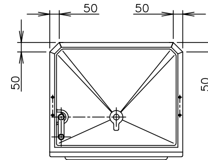
ストッカ上面図
